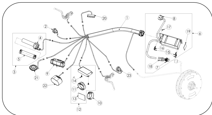
Lámina 9 — INSTALACIÓN 12V Picture 9 — 12V INSTALLATION
