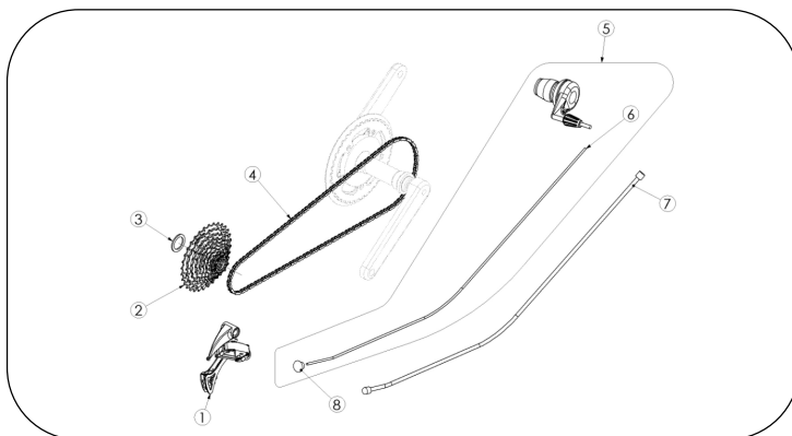
Lámina 10 — TRANSMISIÓN Picture 10 — TRANSMISSION
