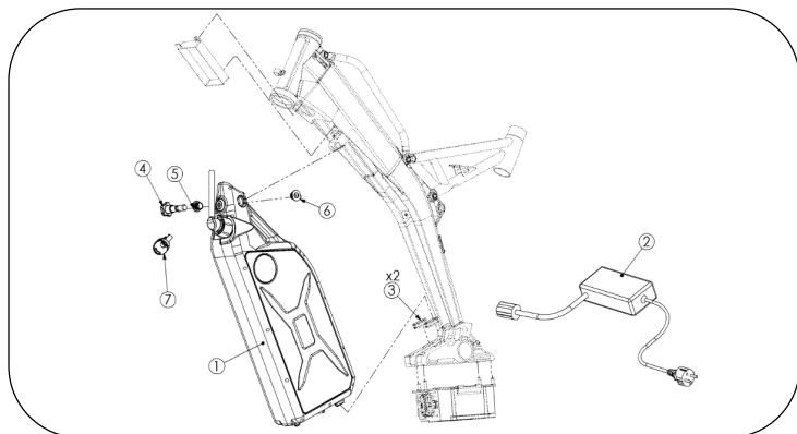
Lámina 11 — BATERÍA DE POTENCIA Picture 11 — POWER BATTERY
